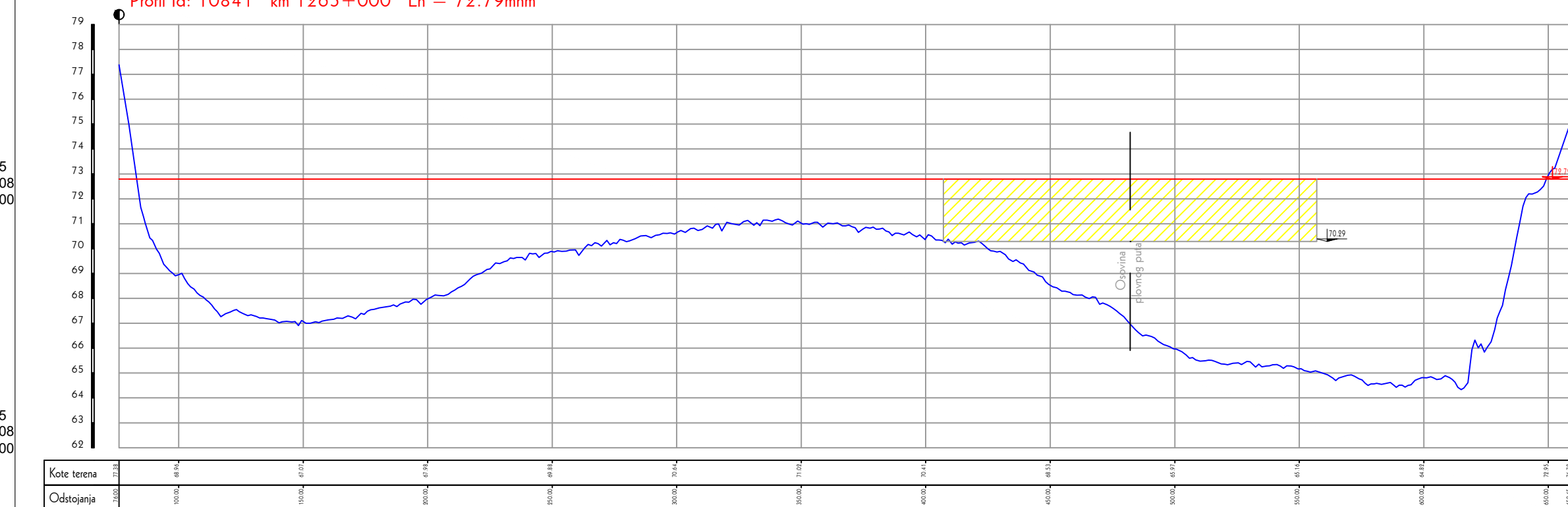
Profil sa najmanjom raspoloživom dubinom u okviru plovnog puta. Reka: Dunav, Sektor: Futog Profil Id: 10841 km 1265+000 En = 72.79mm
